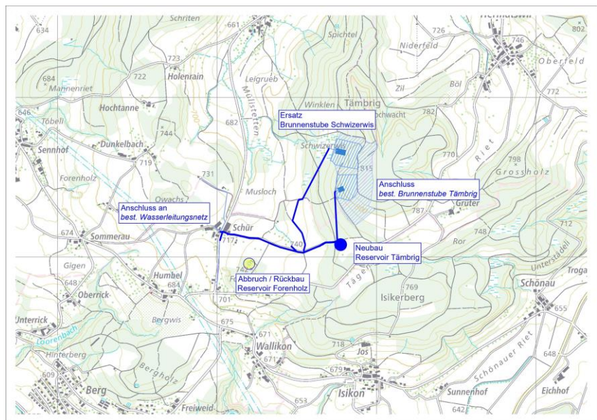
Planausschnitt altes und neues Reservoir inkl. Verbindungsleitungen
